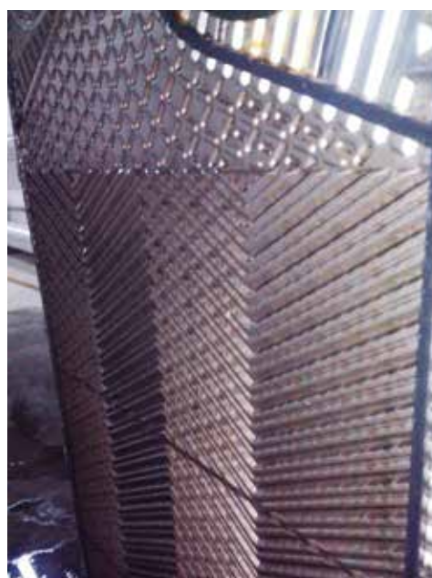
安装S250 四个月, 打开换热板仍保持清洁。
