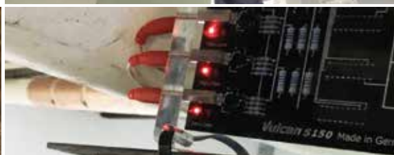
S150设备安装在无尘车间管道上，运用于处理注塑机用水结垢情况
