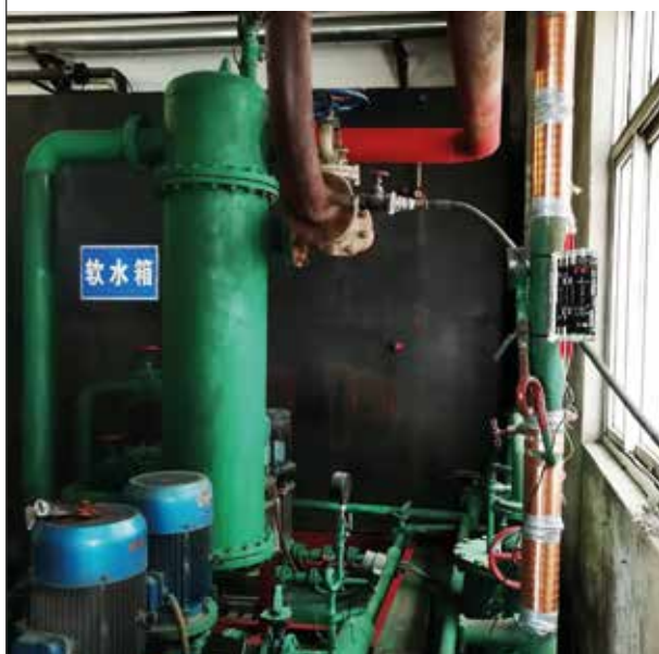
Vulcan S25安装在锅炉房总管道
