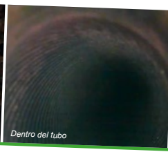
Enfriador del condensador #3 Ø 67 cm. tubo Ø 7/8", longitud: 418 cm
