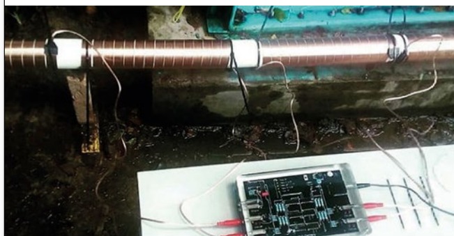
图1. 沃肯(Vulcan)安装在主进水管线上。
