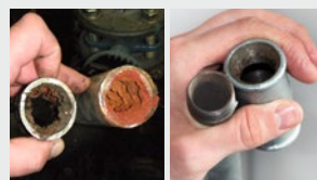
Tuyauterie
