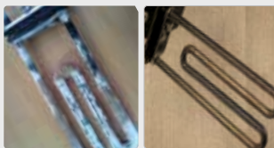
Нагревательный элемент
