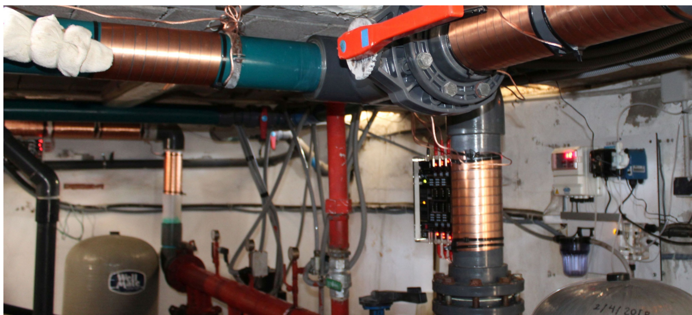
Vulcan S100 au niveau de la conduite d'eau froide (Ø 110 mm) pour 200 appartements et la chaudière
