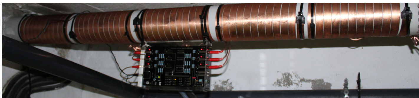
Vulcan S100 au niveau du deuxième tuyau d'eau froide (Ø 110 mm) pour 200 appartements
