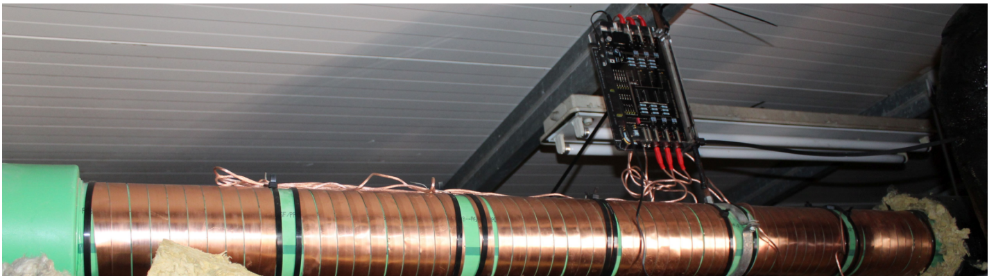
Vulcan S100 En el circuito de agua caliente general Ø 110 mm
