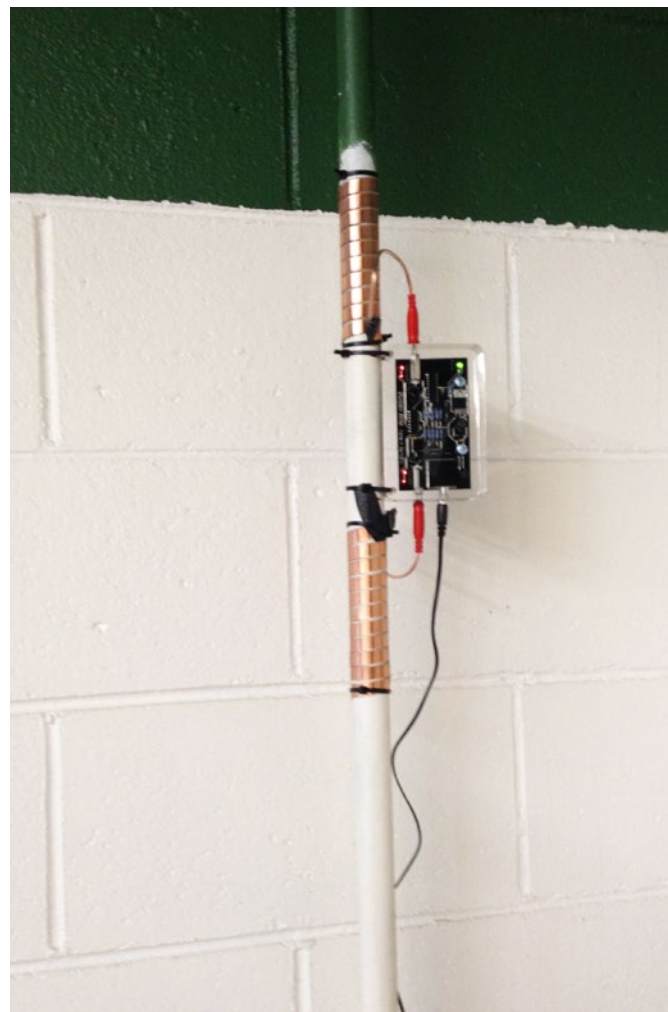
Vulcan S10安装在供水总管上。
