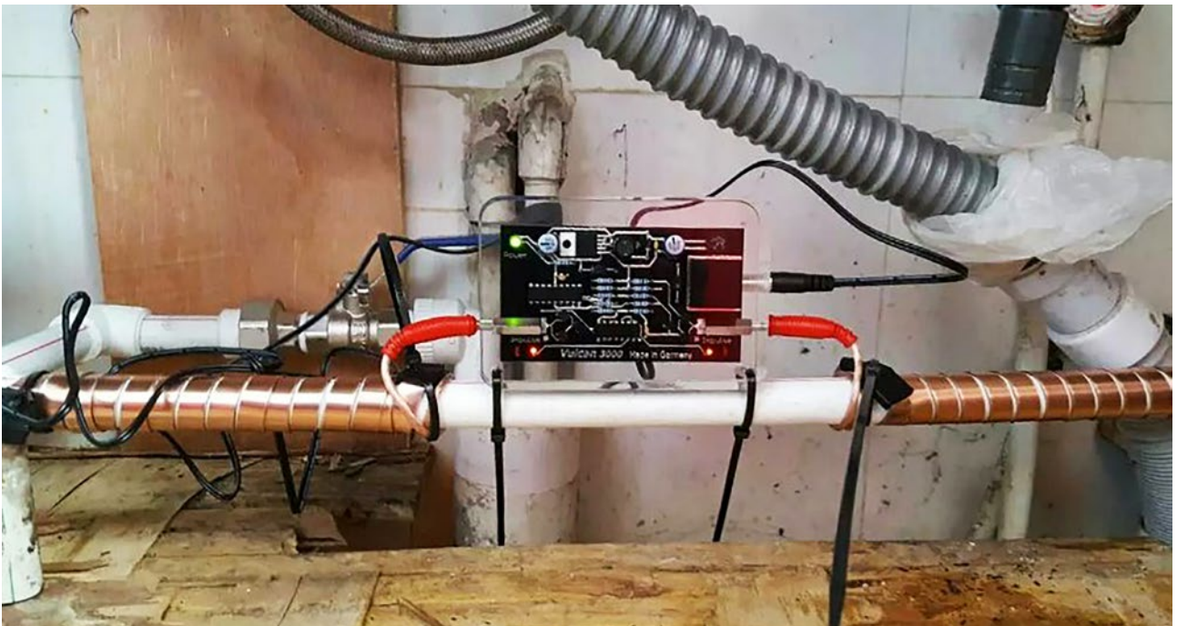
安装在家庭生活用水主管道的沃肯 (Vulcan) 装置 - V3000
