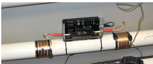
安装在泳池撒沫器主管线上的Vulcan 5000
