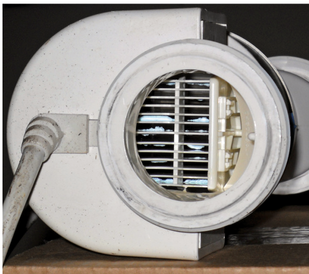
沃肯 (Vulcan) 装置安装30天前, 正在运转的泳池氯化器
