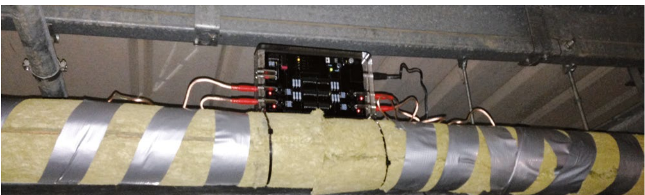
安装Vulcan S25装置时，管道和脉冲电缆外都重新包有绝缘材料
